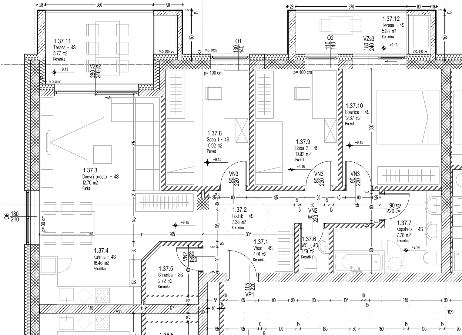
Stanovanje
