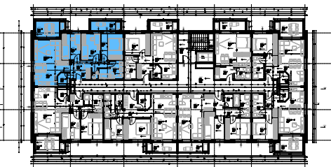
Objekt 1 - 3. nadstropje
