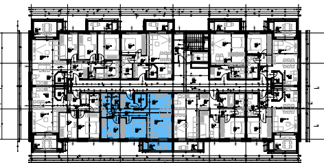
Objekt 1 - 4. nadstropje
