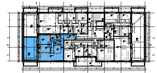
Objekt 1 - 5. nadstropje
