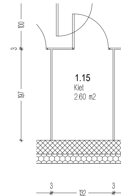
Klet
