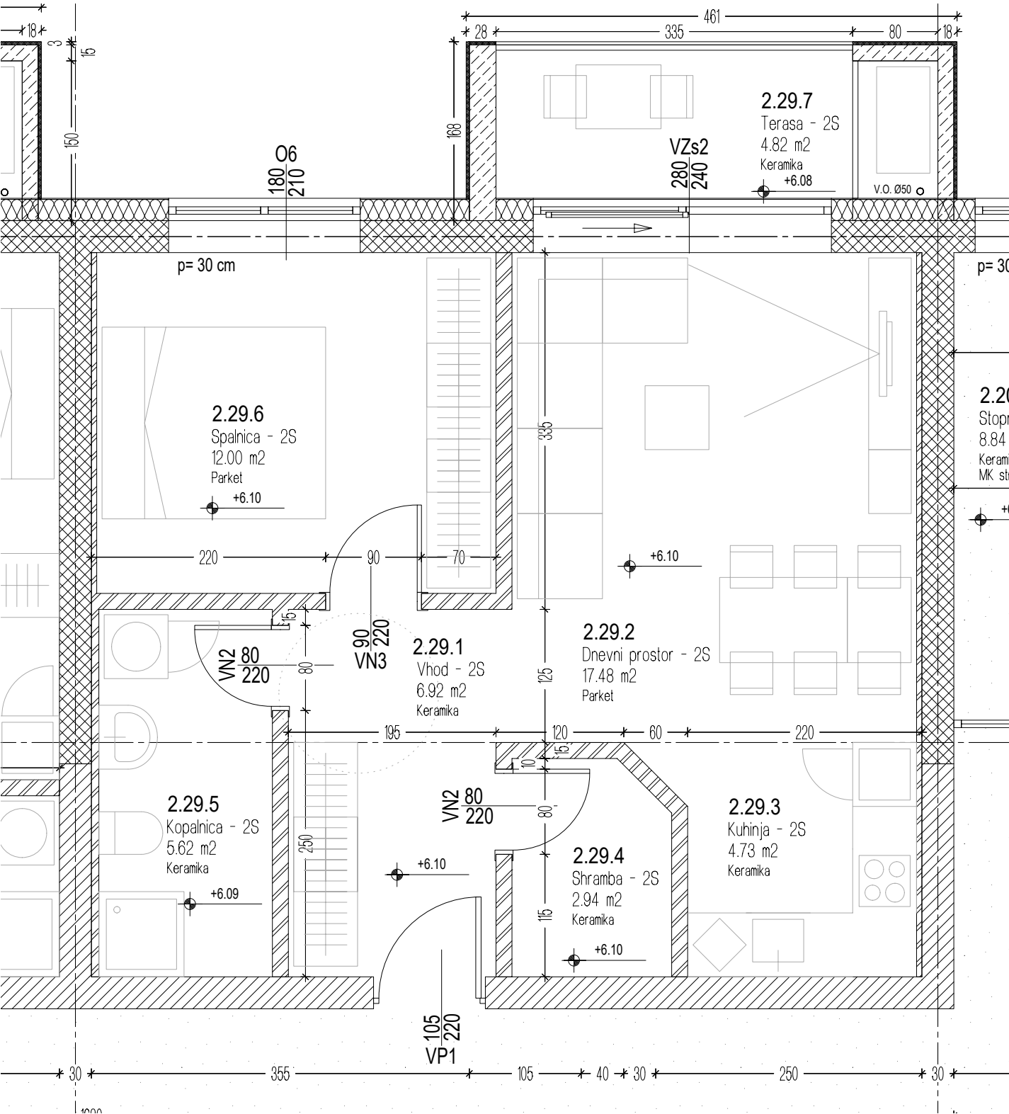
Stanovanje
