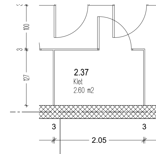
Objekt 2 - 4. nadstropje
