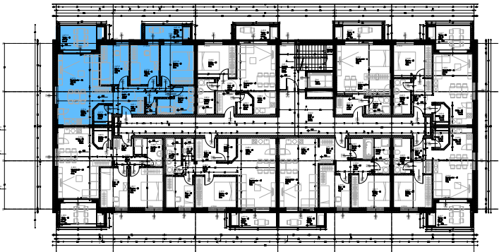
Objekt 2 - 4. nadstropje
