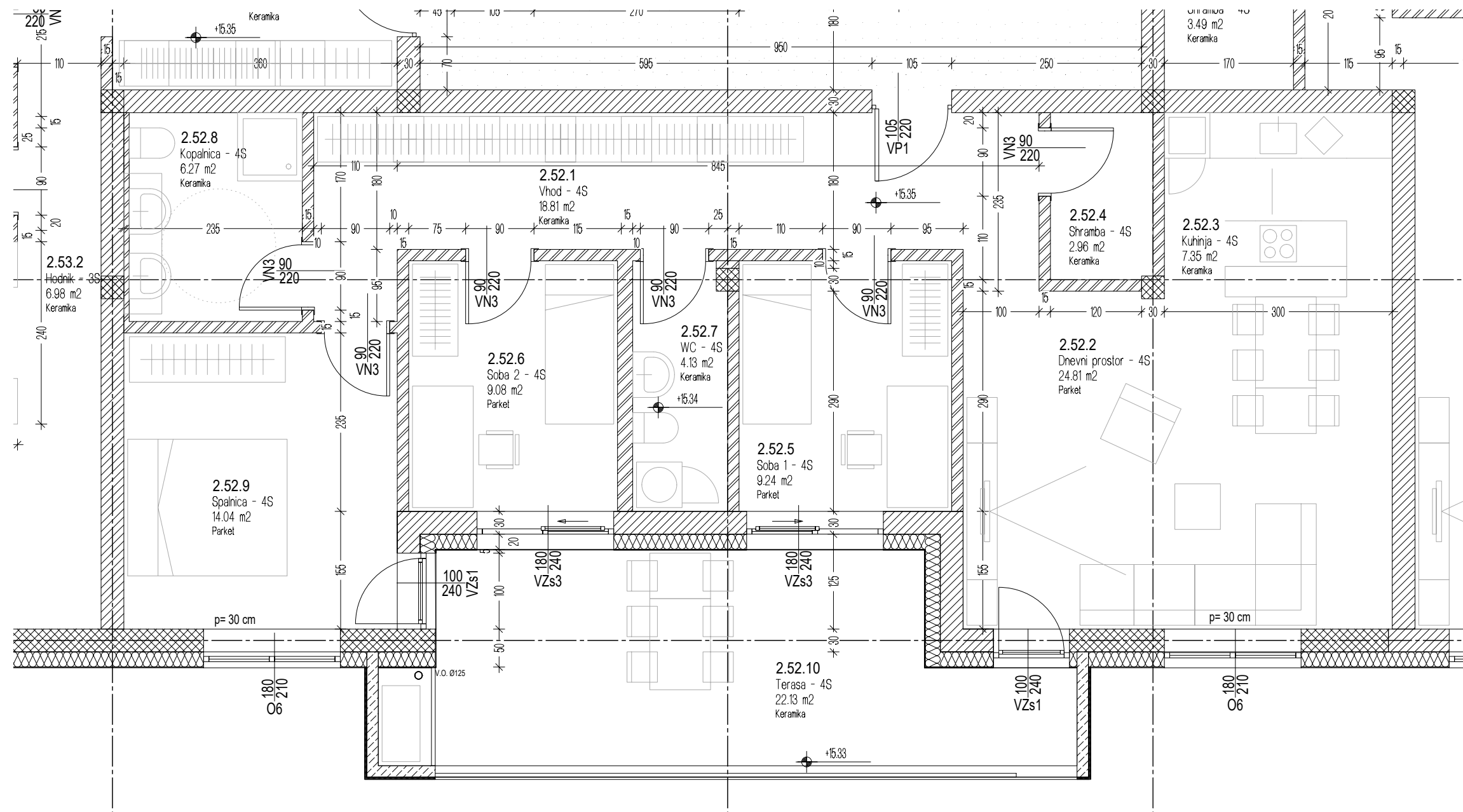
Klet
